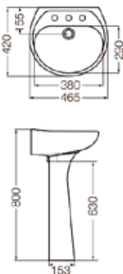
LEA1-B Lavatorio 1 agujero LEA3-B Lavatorio 3 agujeros CTF-B Columna Lavatorio
