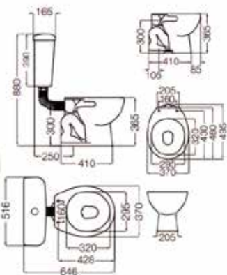
DPCXF-B Depósito de colgar descarga simple 9 lts IFA-B Inodoro corto 9 lts
