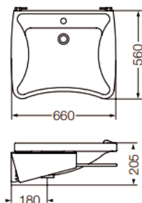
LET1F-B Lavatorio 1 Agujero Soporte Fijo
