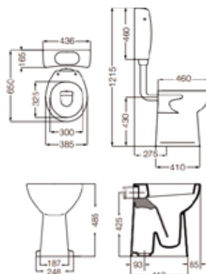
DTE6F-B Depósito de Colgar Descarga Simple 6 Its IETMJ-B Inodoro Corto 6 Its
