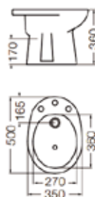
BEA1-B Bidet 1 agujero BEA3-B Bidet 3 agujeros
