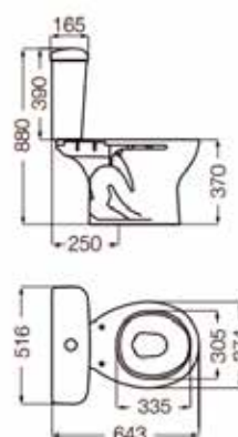
DAS4A-B Depósito de Apoyar descarga simple 4,5 lts IALQ-B Inodoro Largo 4,5 lts.
